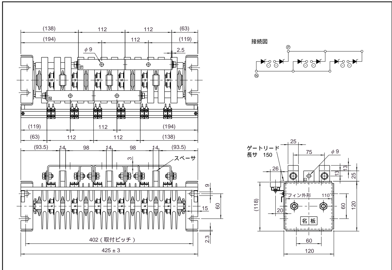
FTS302TG外形図
