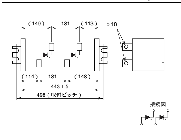
FTS1000CJ, FTS1500CJ外形図
