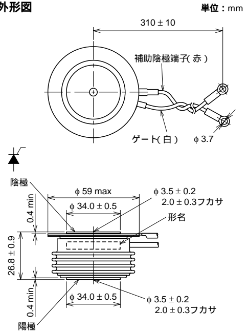
外形図
