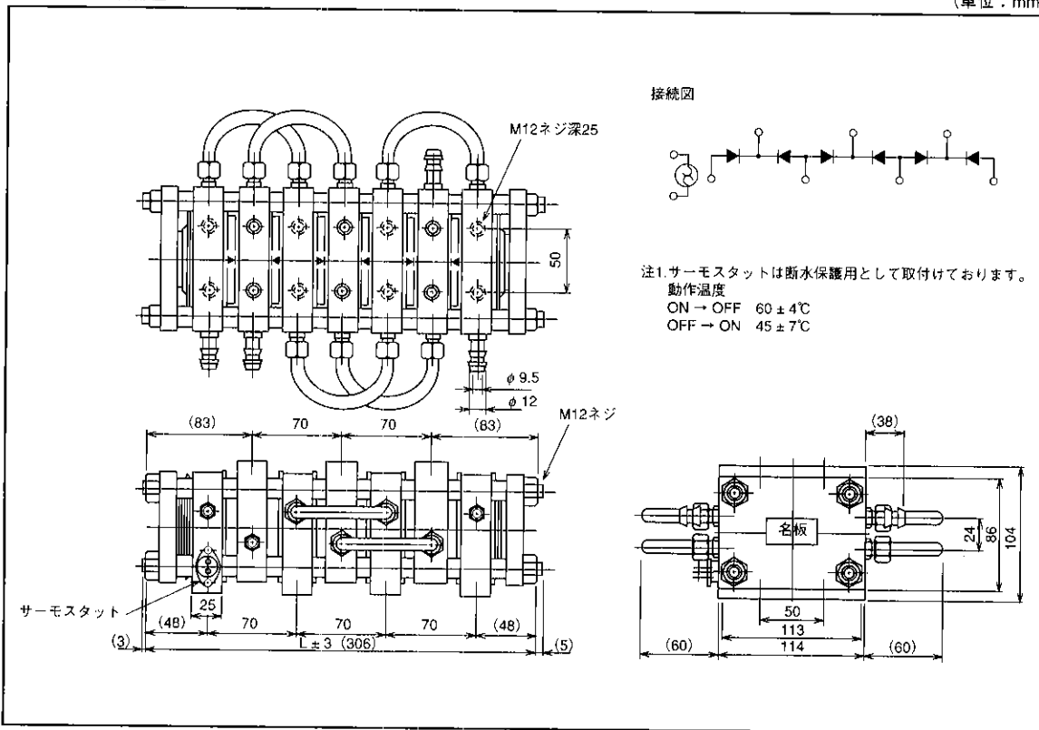
FDS3500H6W外形図
