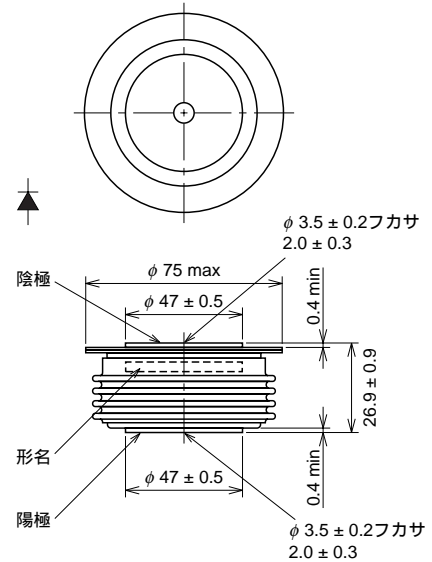
外形図
