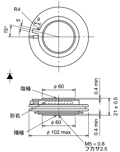
外形図
