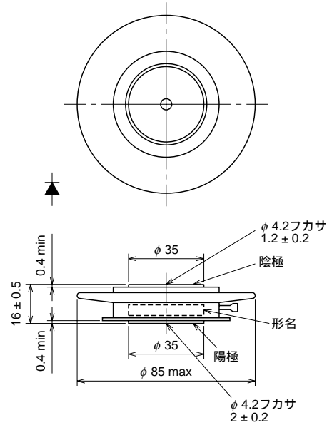
外形図
