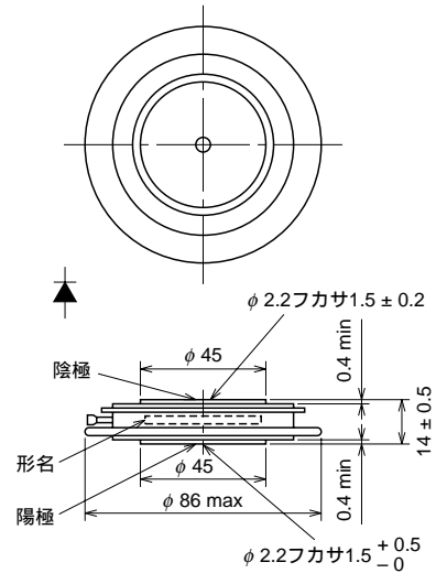
外形図
